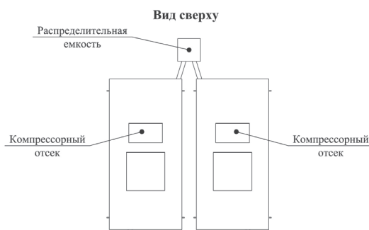
Рис. №11. УОСВ ТОПАС 150 с самотечным отводом очищенной воды
